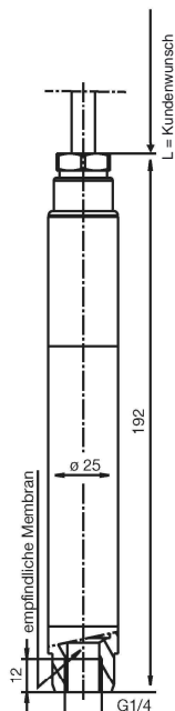
Подключение к процессу 567
