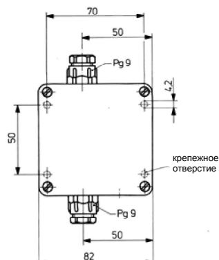
Клеммная коробка с компенсацией давления Артикул №: 40 /00061206
